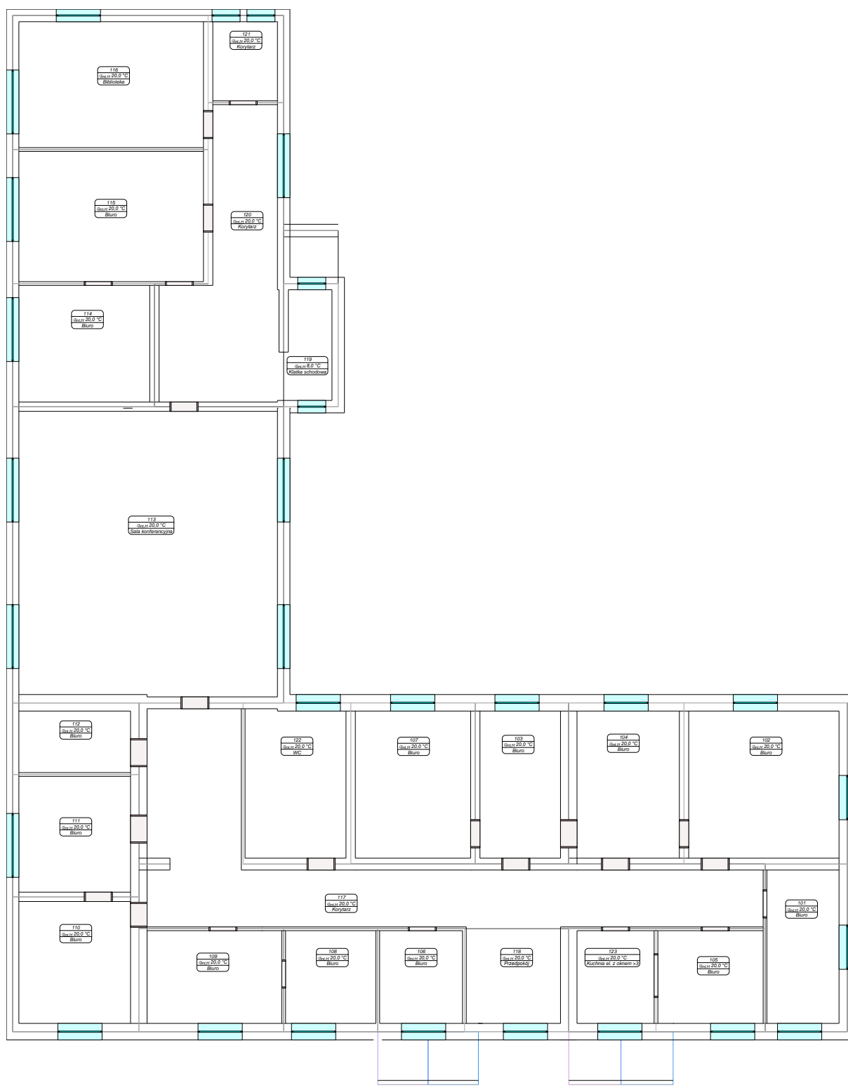
Rzut piętra.
